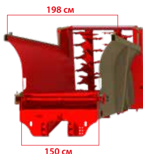
Округленная форма кузова для упрощения выгрузки продукта, реализованная методом гибки для увеличения жесткости стенок.
