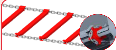
Планки из профилей, приваренные к морским цепям 14 (чтобы избежать накопления продукта) + сваренные приводные звездочки.
