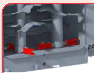
Откидные молотки на износостойком кольце для лучшего измельчения.
