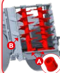
Разбрасывающие валы \varnothing 820 или 900 мм в зависимости от модели, спирали 10 мм.
